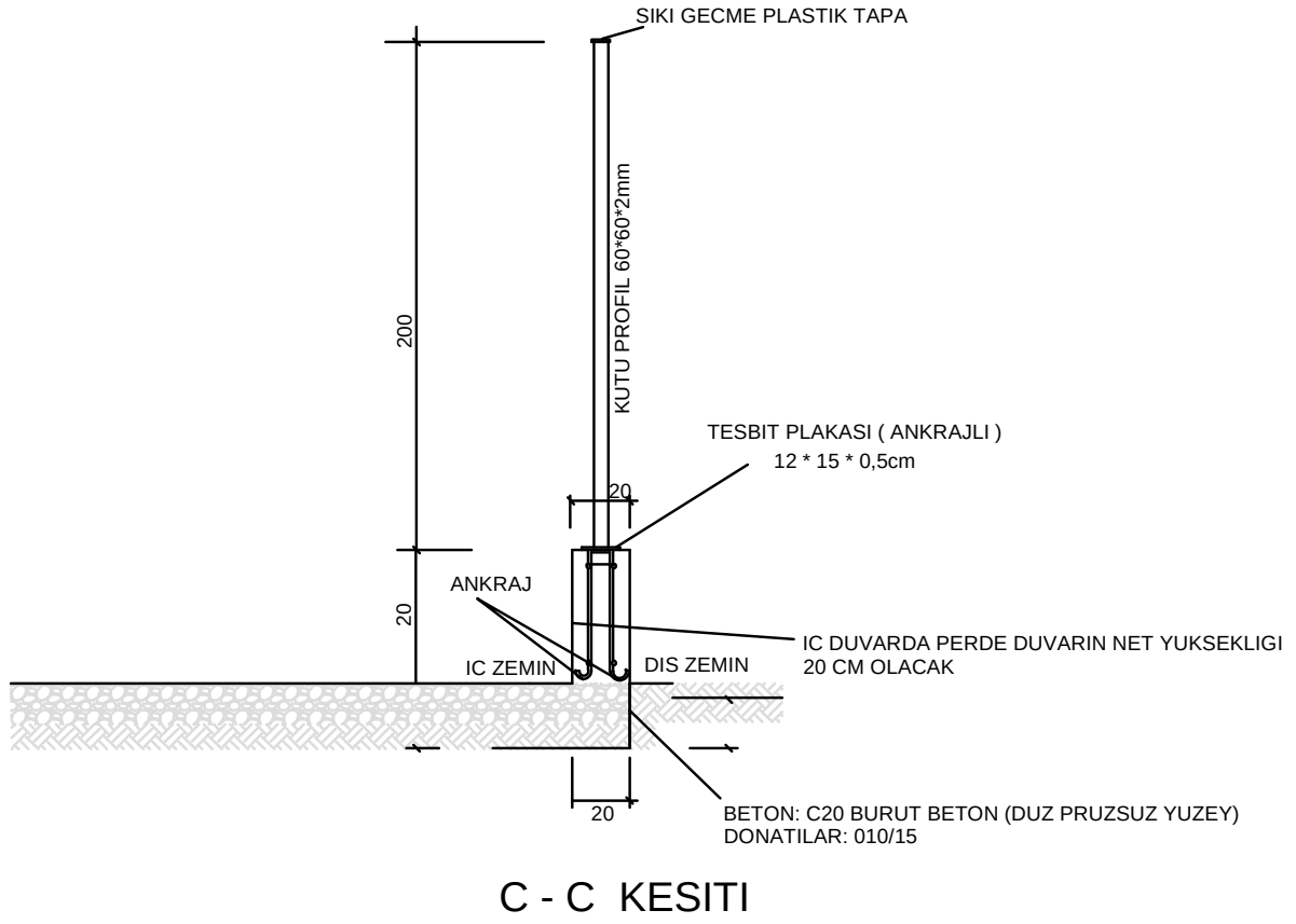
Şekil 2 : MÜŞTERİ İSTASYONU TEL ÇİT KESİT DETAYLARI
